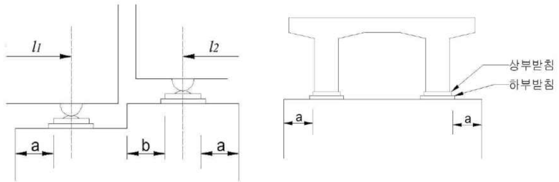
(a) 선로방향 (b) 선로직각방향 【그림 3.2.18】 받침의 끝에서 거더 끝단까지의 거리(a 및 b)의 값
