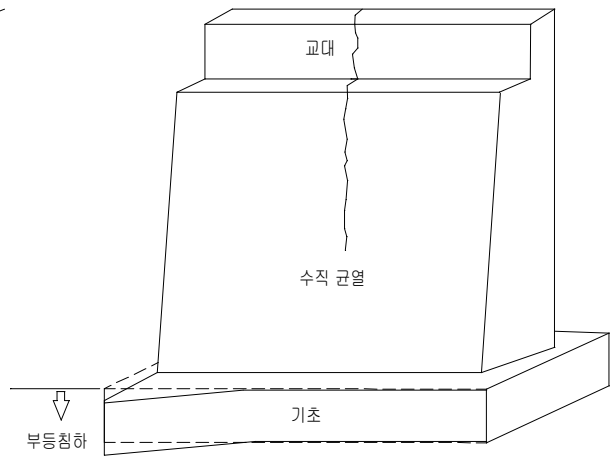
【그림 3.2.10】 부등침하로 인한 교대의 수직균열
